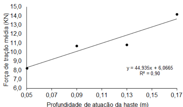
Figura 1 – Força de tração média requerida na barra de tração em função da profundidade de atuação das hastes sulcadoras de adubo.
